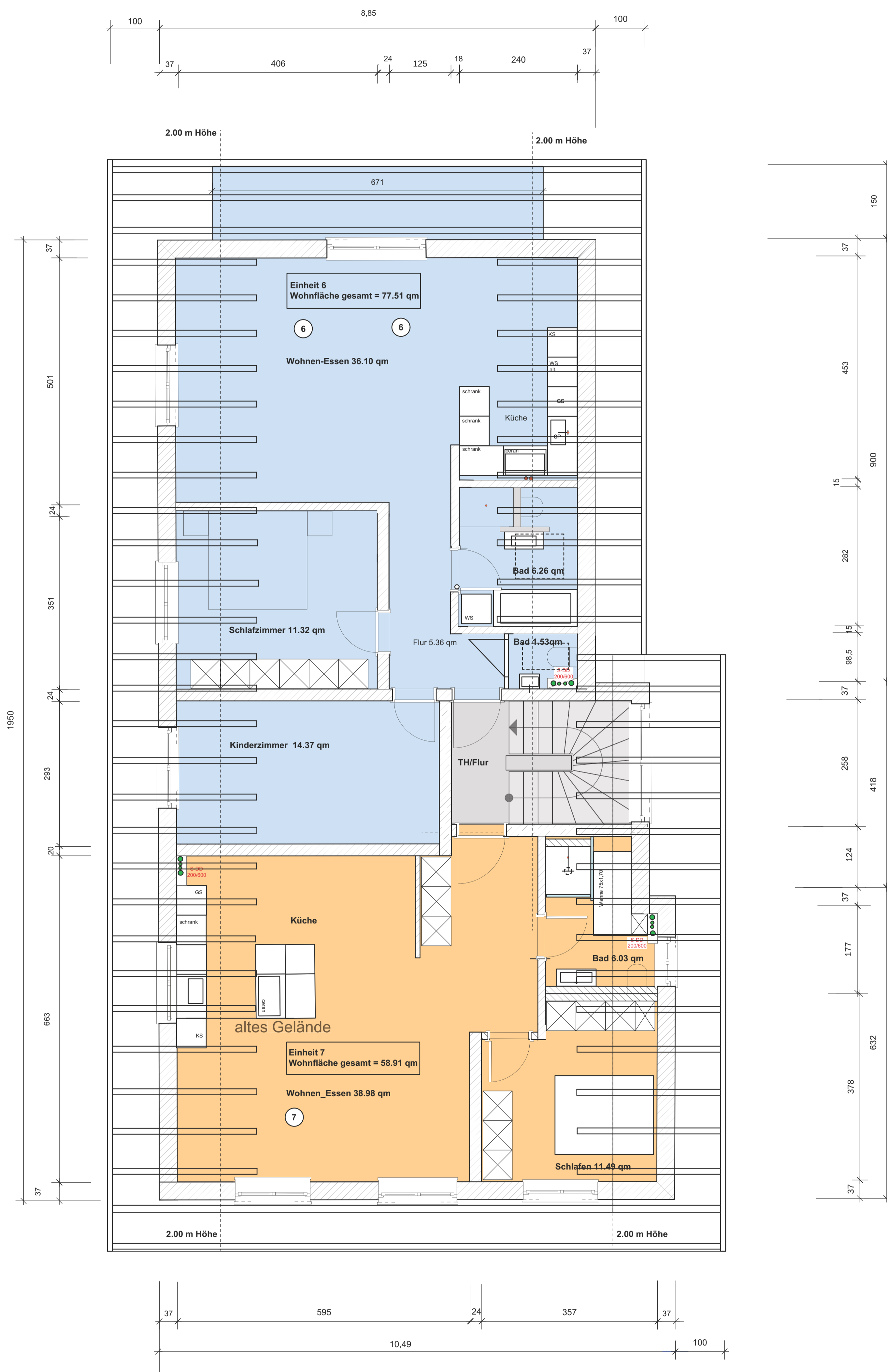
Grundriss Dachgeschoss
