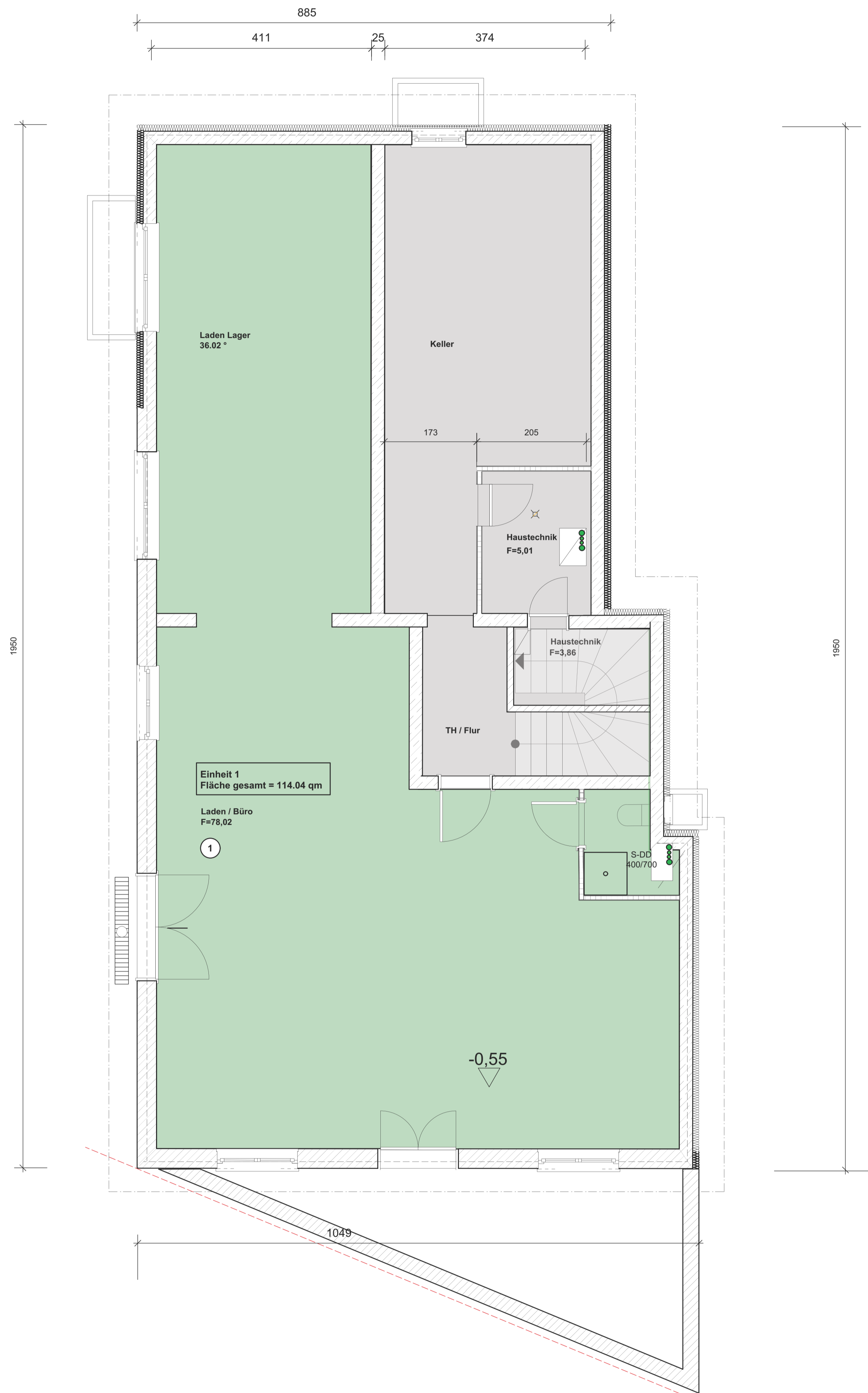
Grundriss Untergeschoss
